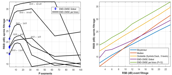
(a) Évolution RSB=f(P) . (b) Comparaisons méthodes.
