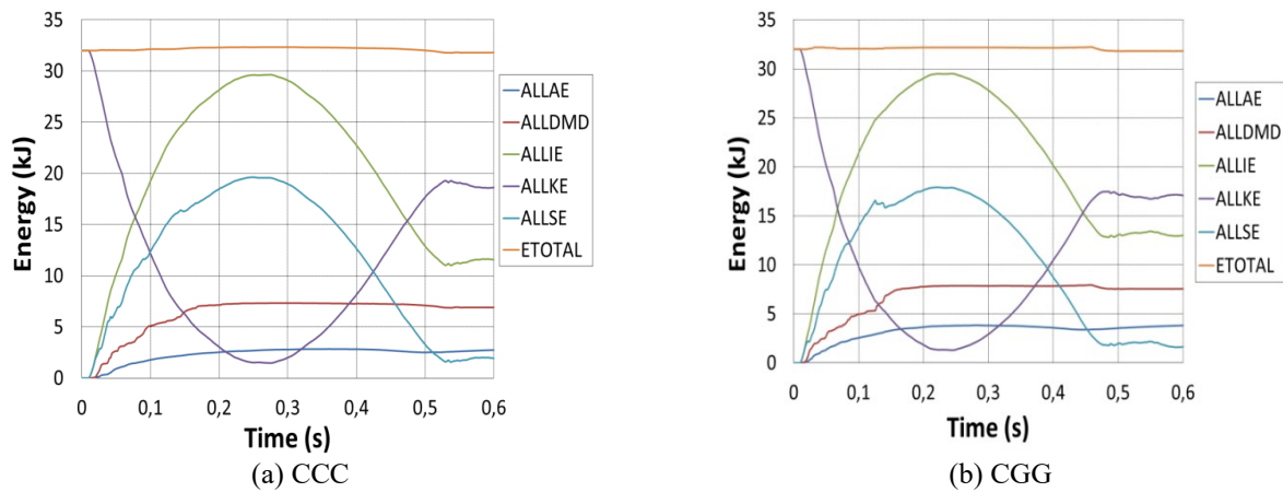
Figure 8. Impact energies versus time ( m=1 tonne, V=8\text{m/s} ).
