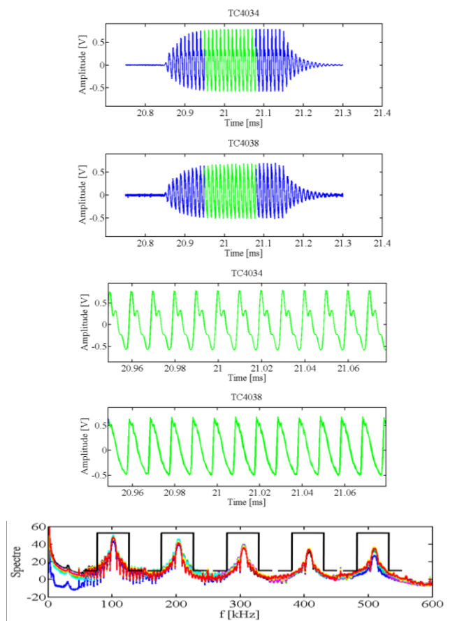
Figure 3 : Signaux temporels acquis avec deux hydrophones. Mesures réalisées au bassin de l'Ifremer (hydrophone TC4034 : bande passante limitée à 500kHz, hydrophone TC4038 : bande passante limitée à 800kHz). De haut en bas : mesures à 41m ; zoom sur le signal (à noter que le signal est déformé avec l'hydrophone TC4034 car seules les 5 premières harmoniques sont mesurées à cause de la bande passante de l'hydrophone) ; spectres typiques mesurés.
