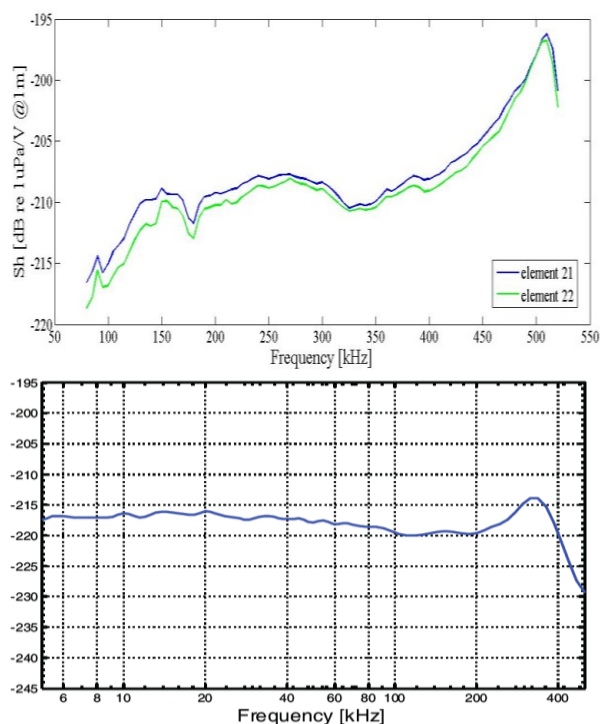
Figure 5 : Sonde constituée de céramiques sciées avec backing en air. En haut : sensibilité obtenue. En bas : sensibilité de l'hydrophone Reson TC4034.
