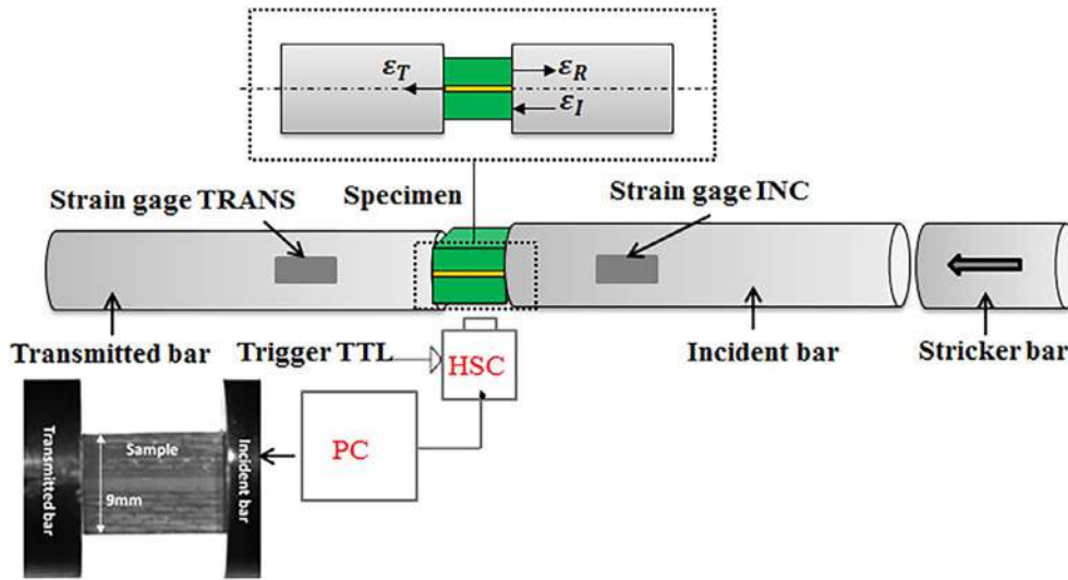
Fig. 2. Split Hopkinson bar apparatus.
