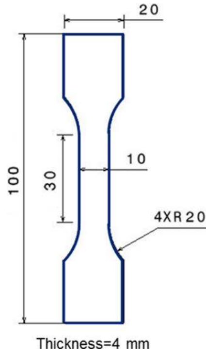
Fig. 2 Tensile specimen
