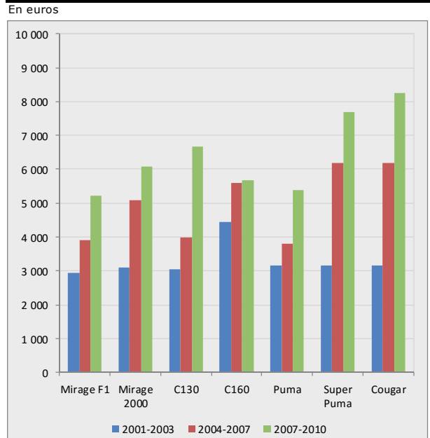
Figure 2 : Crédits d'Entretien Programmé des Matériels à l'heure de vol des avions de l'armée de l'air
