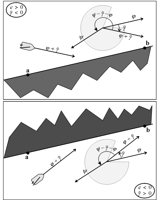
Fig. 9. En haut, le robot est au dessus de sa ligne ( e > 0 ) et le cap \varphi + \bar{\gamma} est tenable car il est dans le secteur gris. En bas, e < 0 et le cap n'est plus tenable.
